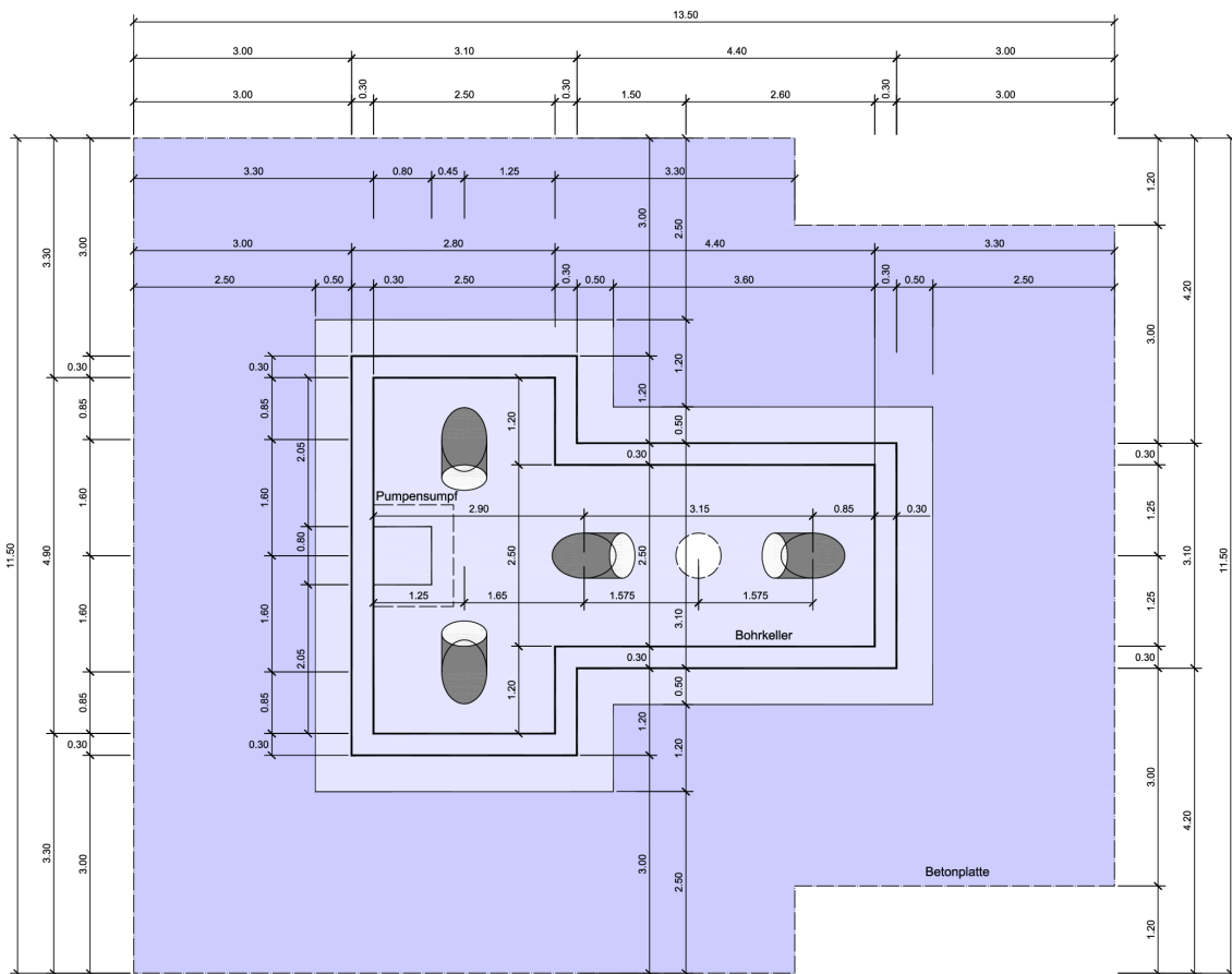
Fig. 5.3: Grundriss des Bohrkellers für fünf Bohrichtungen.
