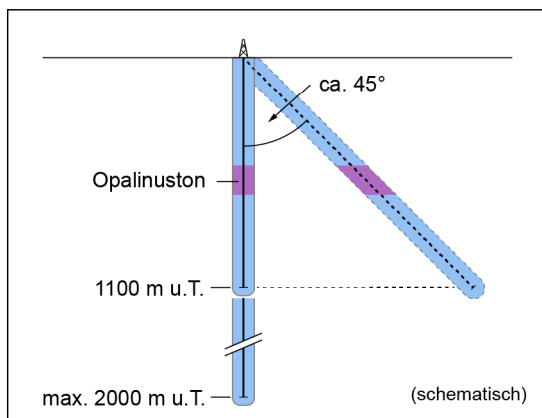
Fig. 7.1: Lage und Ausdehnung der möglichen Bohrfade der Sondierbohrungen Uhwiesen in Bezug auf den SMA-Lagerperimeter mit Sicherheitsabstand von r = 50 m um die potenziellen Bohrfade.
