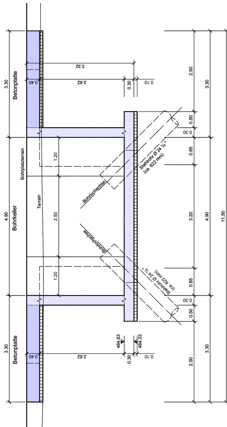
Fig. 5.5: Querschnitt des Bohrkellers (A-A) mit den Bohrrichtungen Nordost und Südwest und den entsprechenden Bohransatzpunkten (Lage des Schnitts vgl. Beilage 8).
