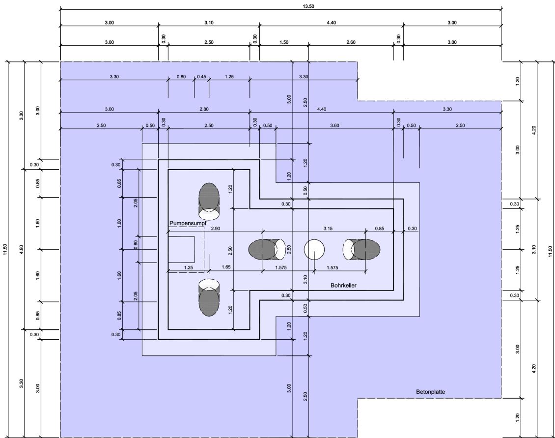
Fig. 5.3: Grundriss des Bohrkers für fünf Bohrrichtungen.
